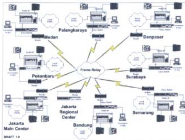
Gambar 2 : Sistem Pengiriman Data
